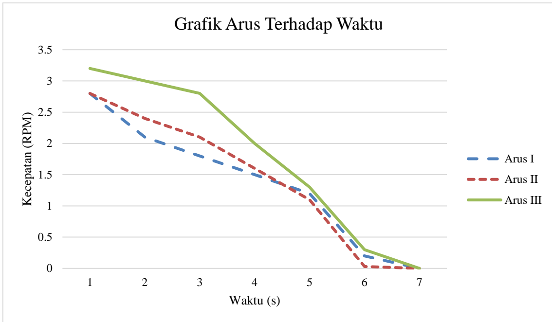
Gambar 1 Grafik Arus Terhadap Waktu - (600 rpm – 3.75 kg)
