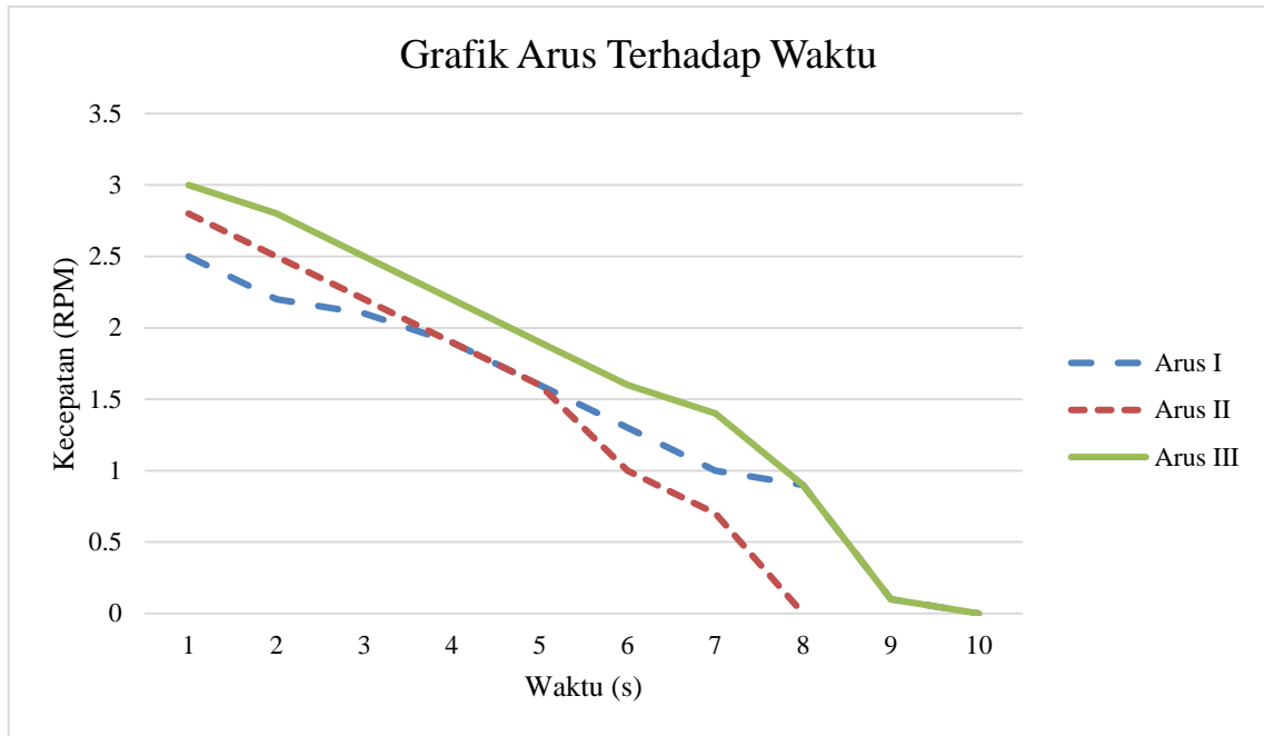
Gambar 58. Grafik Arus Terhadap Waktu - (600 rpm – 5 kg)
