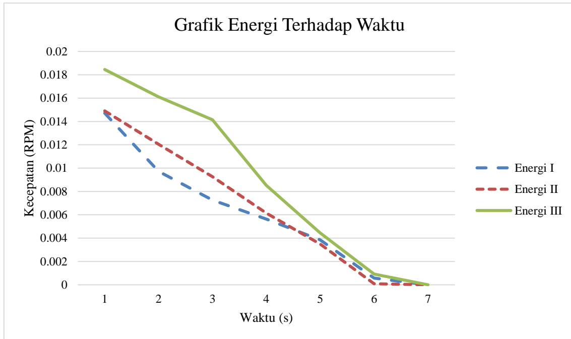
Gambar 25. Grafik Energi Terhadap Waktu - (600 rpm – 3.75 kg)
