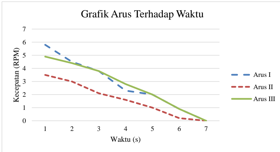
Gambar 18. Grafik Arus Terhadap Waktu - (800 rpm - 2.5 kg)
