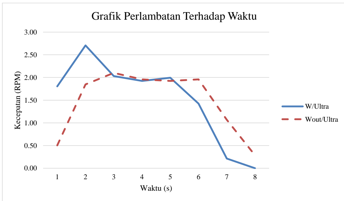
Gambar 22. Grafik Perlambatan Terhadap Waktu - (600 rpm - 2.5 kg)
