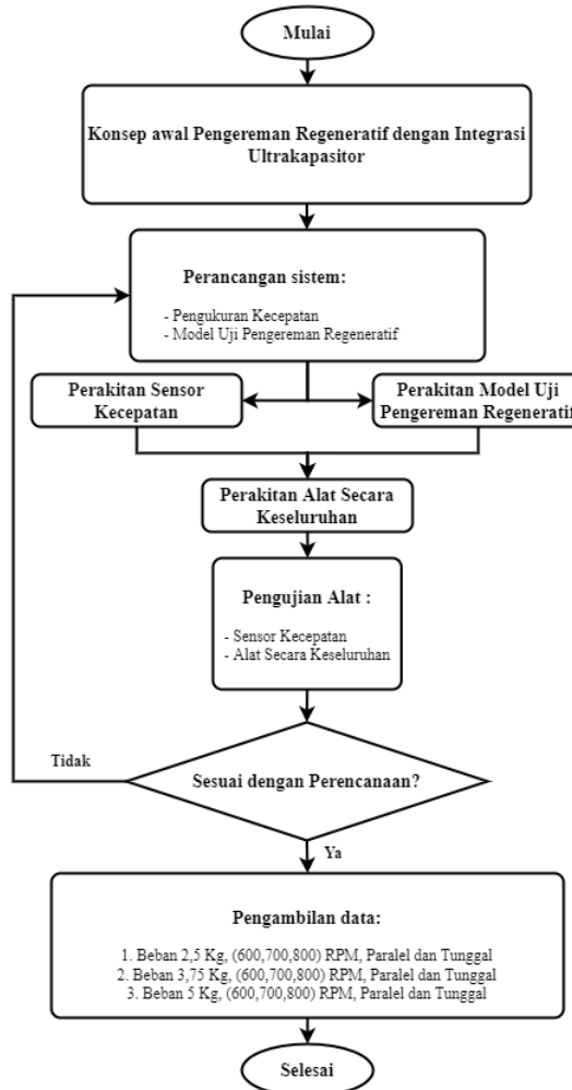
Gambar 1. Diagram kerja alat
